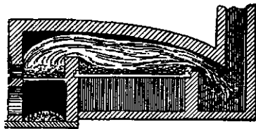
ציור 11. תנור-להב (פירוס)
