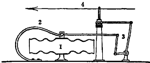
ציור 3. אנרואיד (וידי) (כספה) 1. קופסה; 2. קפיץ; 3. מערכת-מנופים; 4. מחוג
