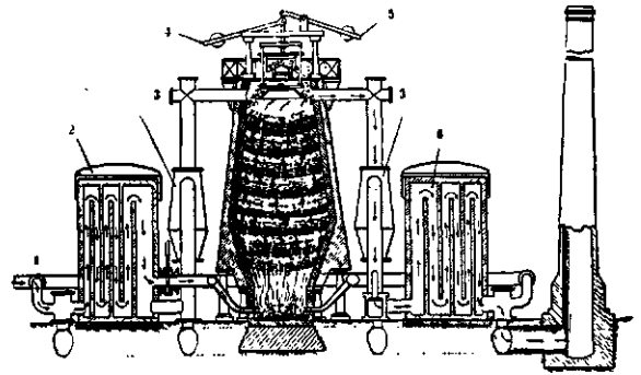
ציור 10. תנור רם (סכמה)
