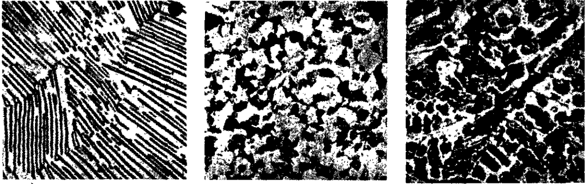
ציור 8. מיקרוצילומים של המבנה של סוגי ברזל ופלדה. א. ב"נפחים לבן: בהיר—צ'קנטיט, כהה—פ'רליט ( 100\times ); ב. פלדה, 0.2% פחמן: בהיר—פ'רליט, כהה—פ'רליט ( 100\times ); ג. פלדה אוקטטית (פ'רליט): שכבות פ'רליט וצ'קנטיט ( 1,000\times ).
