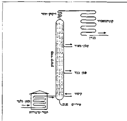
הפקת בנזין ע"י זיקוק ישיר של שמן-ארמה (סכסח)
