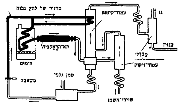
סקמה של מערכת-פיצוח
