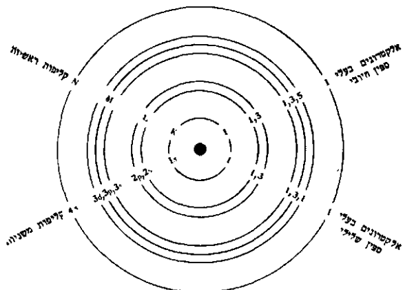
ציור 3. המבנה האלקטרוני של אטום-הברזל החפשי
