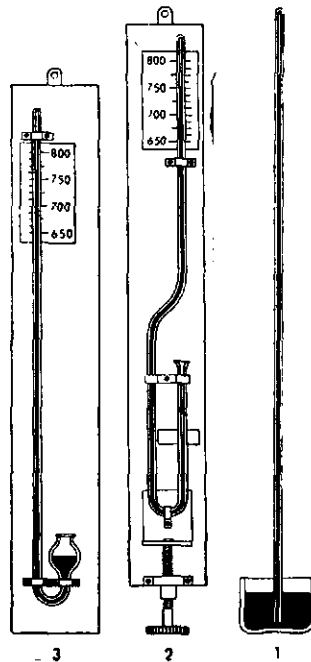
ציור 2. בארומטרים של כספית: 1. ריקטוריצ'לי; 2. בי-גשמה; 3. בבוק.
